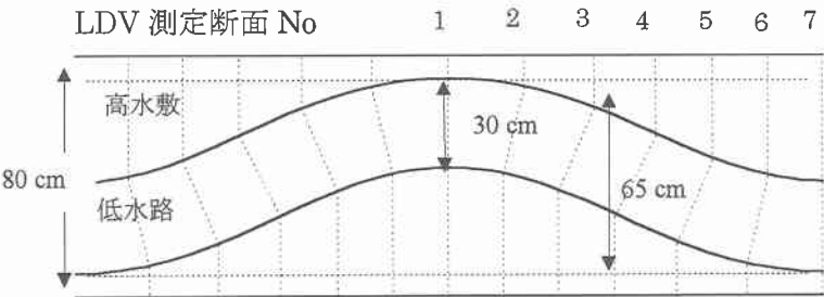
図-2 水路諸元及び測定断面
