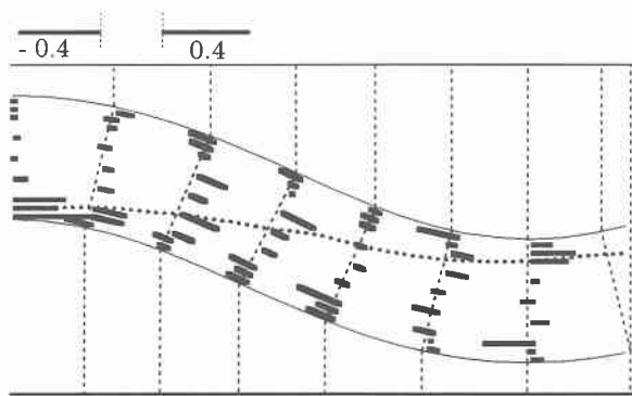
図-4 \tau'_{exe} - \tau'_{ana} の分布 (Dr=0.44)
