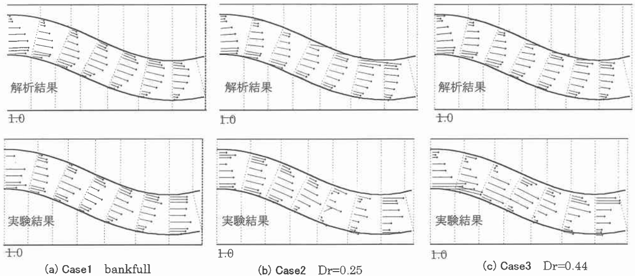
図-3 無次元せん断応力分布の比較
