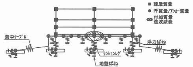
図-4 地震応答解析モデル図
