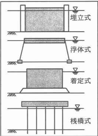
図-1 海洋構造物の工法分類
