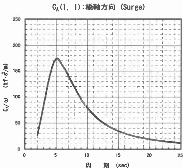
図-2 造波減衰係数 (surge)
