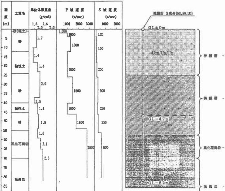
図-2 大州の鉛直アレー
