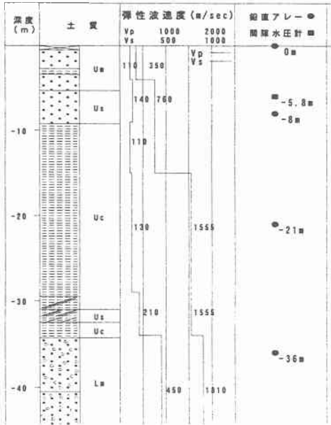
図-1 消防航空隊基地の鉛直アレー 4)
