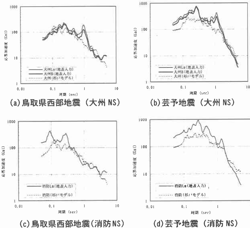
図-4 工学的基盤からの入射波の加速度応答スペクトル
