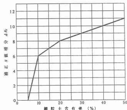
図-1 細粒分含有率と補正 N 値増分 \Delta N_f の関係
