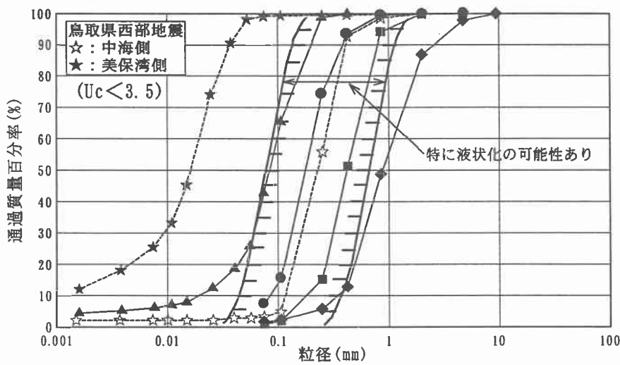
図一 2 噴砂の粒径加積曲線
