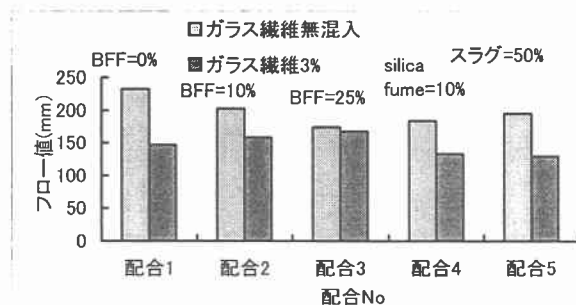
図1 モルタルの流動性
