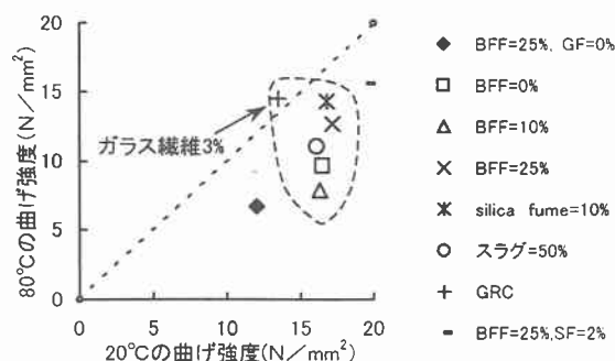
図 4 80℃熱水養生による曲げ強度の低下
