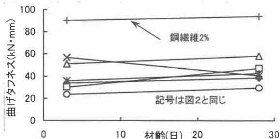
図3 繊維補強モルタルの曲げタフネス
