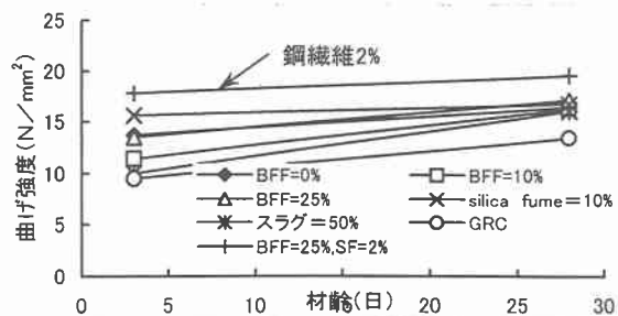
図2 繊維補強モルタルの曲げ強度
