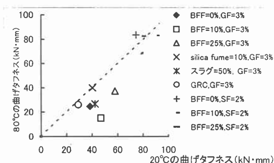
図 5 80℃熱水養生による曲げタフネスの低下
