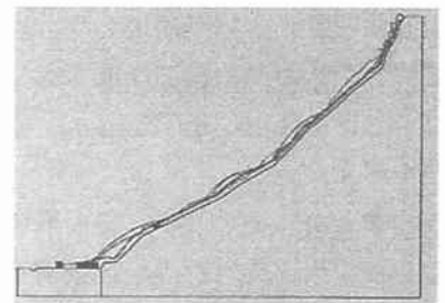
図-1 溝口町の落石軌跡図
