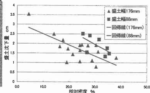
図6 相対密度と沈下量の関係
