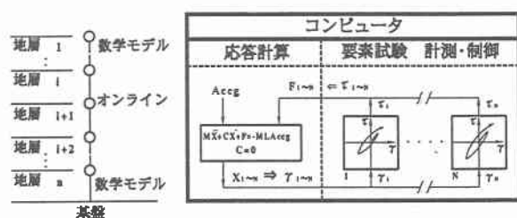
図-1 オンライン地震応答実験手法の概念図
