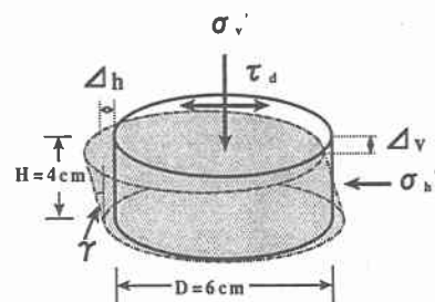
図-3 シェイクダウンモードにおける供試体の状態
