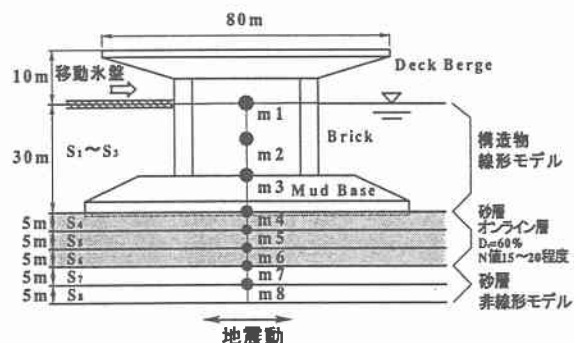
図-2 実験対象モデル図
