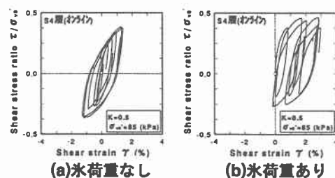
図-5 せん断応力比-せん断ひずみ関係
