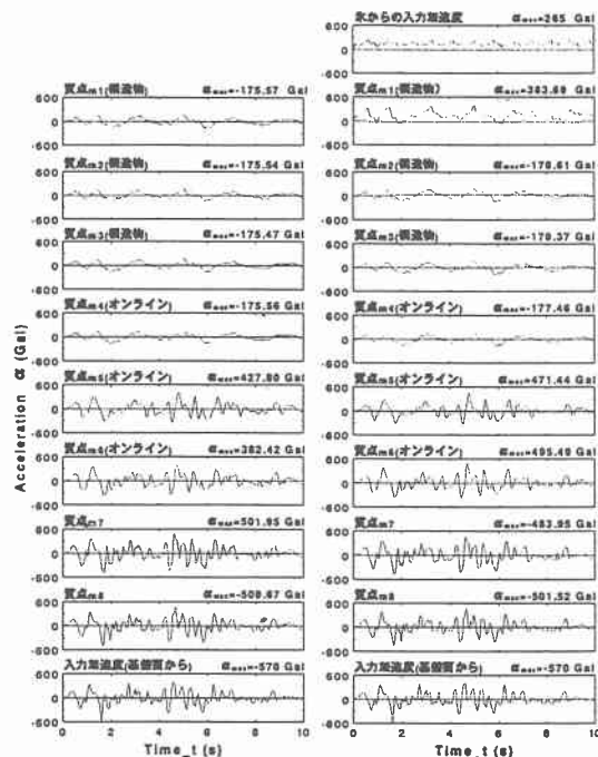
図-4 応答加速度の時刻歴
