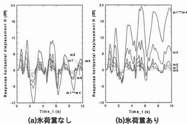
図-7 水平応答変位の時刻歴
