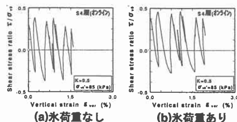
図-6 せん断応力比-鉛直ひずみ関係
