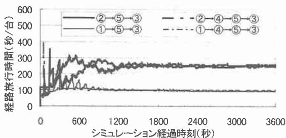
Fig. 4 等時間原則の確認
