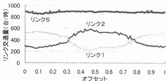
Fig. 3 リンク交通量とオフセット
