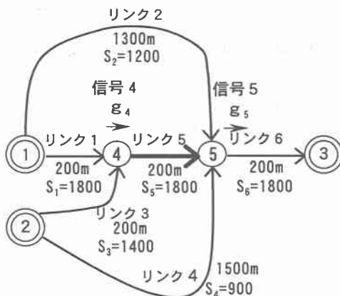
Fig. 1 計算対象ネットワーク
