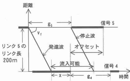
Fig. 2 オフセットによる交差道路の優先度 x
