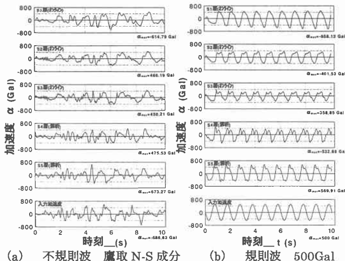
図-4 入力加速度と応答加速度の時刻歴
