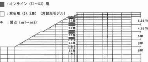
図-2 解析対象モデル図
