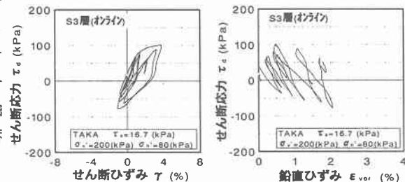
図-5 せん断応力-ひずみ関係（鉛直、側方）
