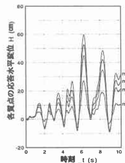
図-6 応答水平変位の時刻歴
