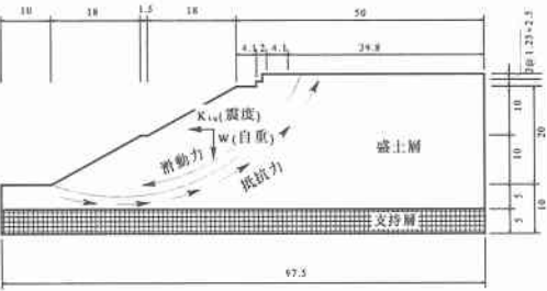
図-2 高盛土のモデル図
