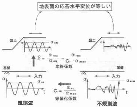
図-1 等価震度の算出フロー
