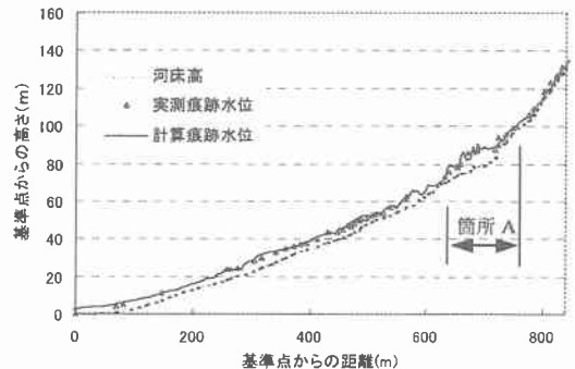
図-4 痕跡水位計算結果
