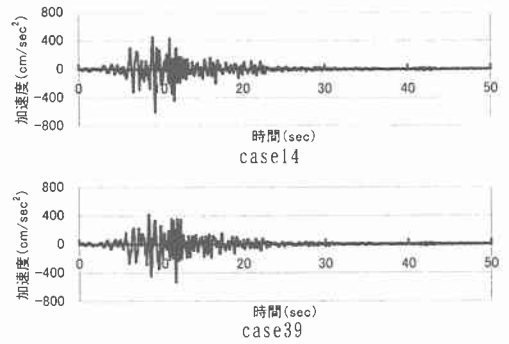
図-6 入力地震動の時刻歴波形
