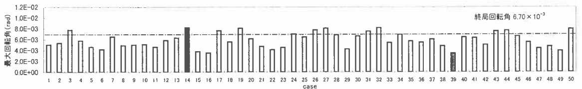
図-3 橋脚基部の塑性ヒンジ部に生じる最大回転角
