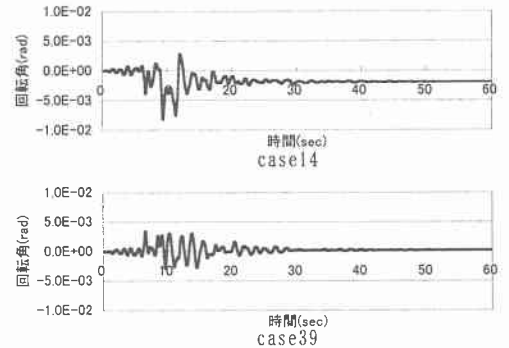
図-7 P2 橋脚の回転角の時刻歴応答波形
