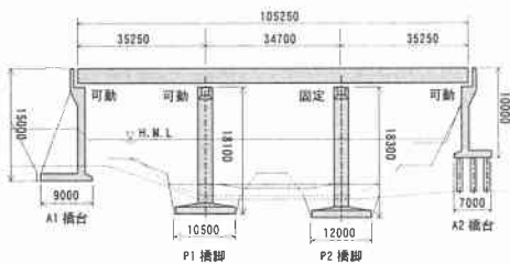
図-1 対象橋梁一般図
