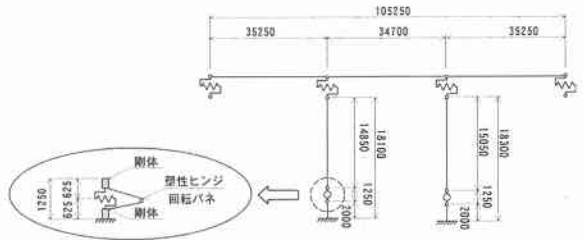
図-2 動的解析モデル
