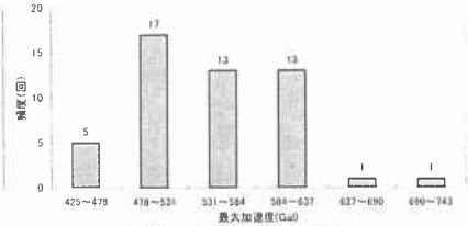
図-5 入力地震動の最大加速度の分布
