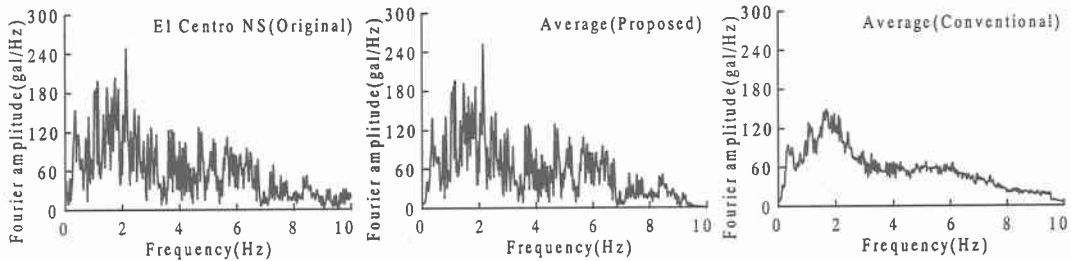
図-2 EL Centro NSのフーリエスペクトル；本法と従来法による模擬地震動各20波の同スペクトルの平均値
