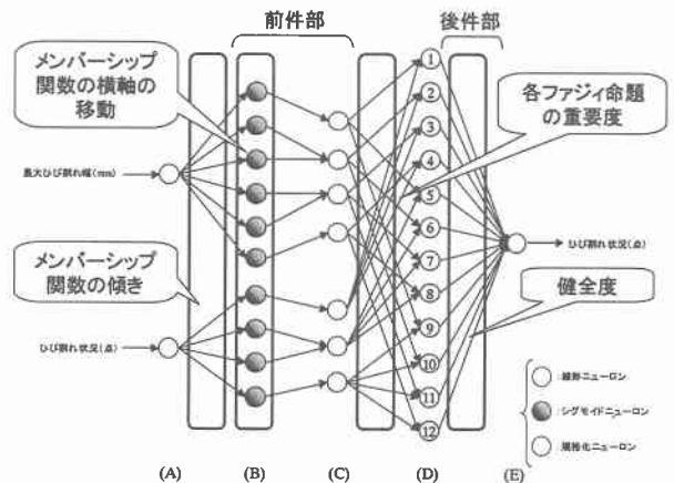
図2 学習により更新されるニューロン
