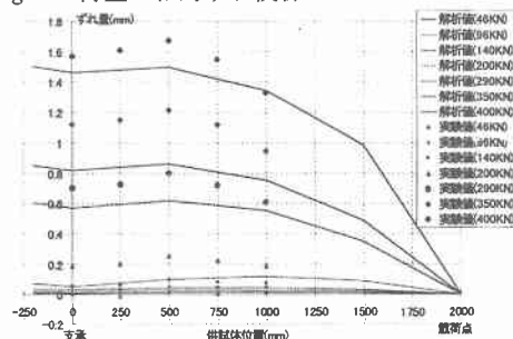
Fig.6 ずれ分布
