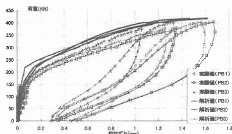
Fig.5 荷重-相対ずれ関係
