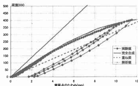
Fig.4 荷重-たわみ関係
