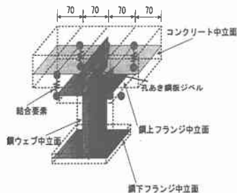
Fig. 3 解析モデル
