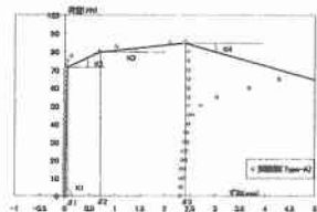
Fig. 1 荷重-ずれ関係
