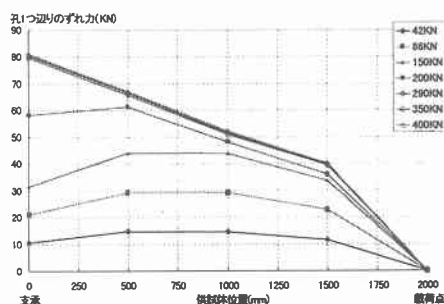
Fig.7 ずれ力分布
