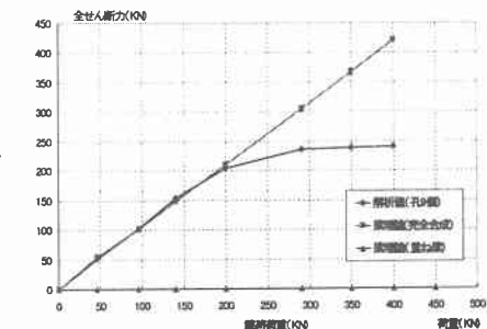
Fig.8 全せん断力-載荷荷重関係
