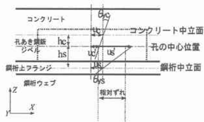
Fig. 2 孔の位置における相対ずれ
