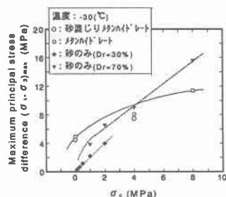
図-3 拘束圧～最大主応力差関係
