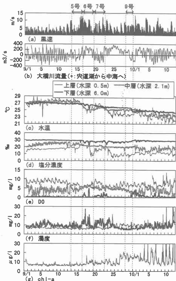
図-4 中海湖心における風速、水温、塩分濃度、DO、濁度、Chl-a 及び大橋川流量 (1998/9/1~10/12)
