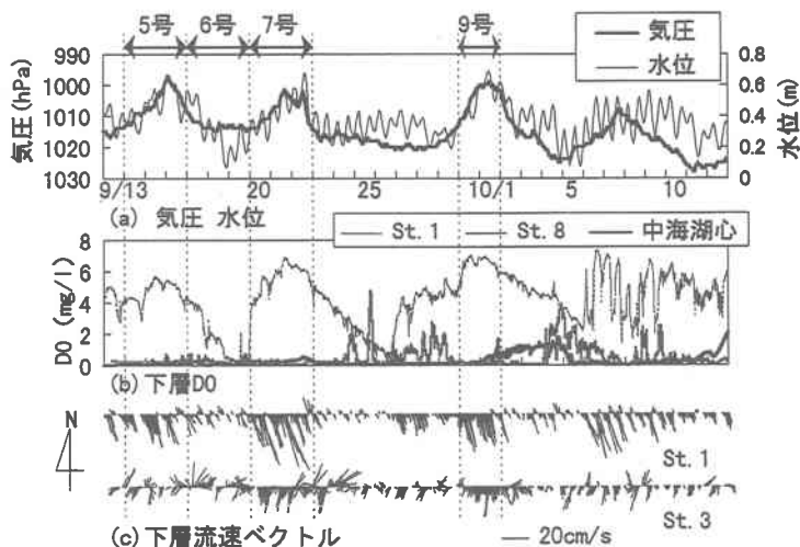
図-2 中海湖心気圧、外海水位、St.1, St.8, 中海湖心における下層 DO 及び St.1, St.3 における下層流速ベクトル
