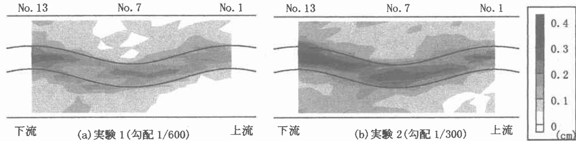
図-1 水面変動振幅コンター
