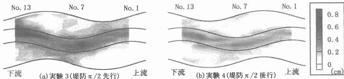
図-3 水面変動振幅コンター
