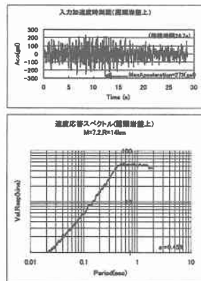
図-3 模擬地震動
