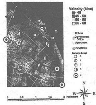
図-6 被害と速度分布
