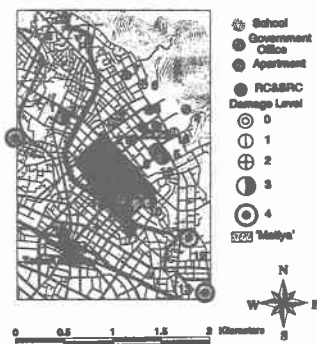
図-2 被害分布
