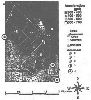
図-5 被害と加速度分布
