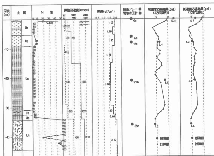
図-4 鉛直アレー観測点での地中最大加速度分布の比較
