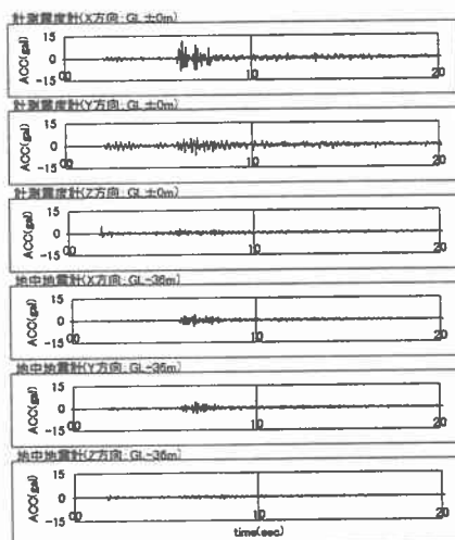
図-3 地表と地中の加速度記録
