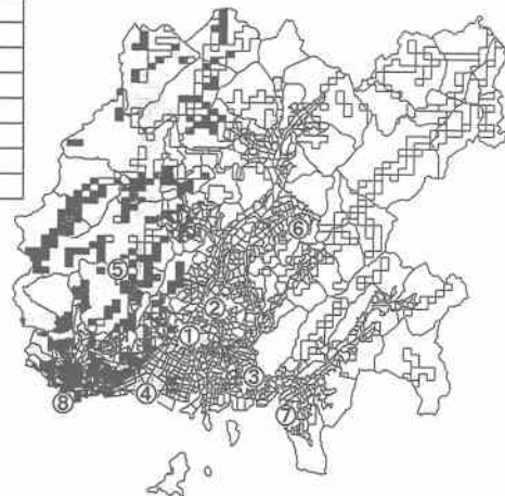
図-2 地震観測位置と最大加速度予測分布
