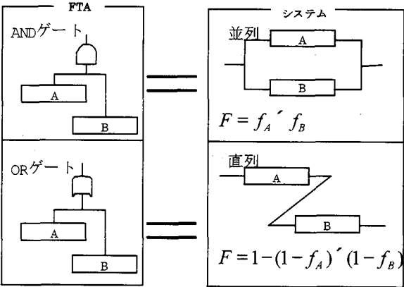
図-1 論理記号の系統的観点
