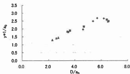
図4 液状化深さ(1)
