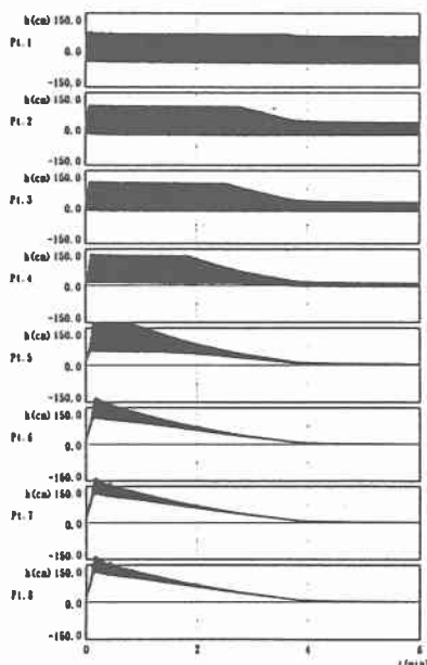
図2 変動間隙水圧図
