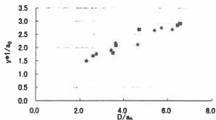
図5 液状化深さ(2)
