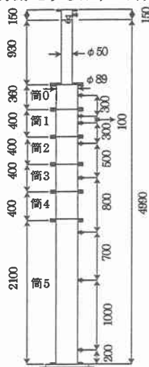
図1 試料容器 (mm)
