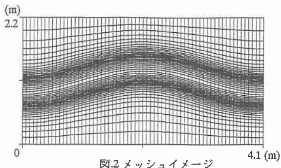
図2 メッシュイメージ
