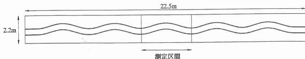
図.1 実験水路
