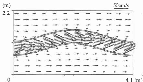
図4 流速ベクトル図（計算） 実線：高水敷高さより上 破線：高水敷高さより下
