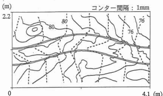
図5 水位コンター 実線：実験 破線：計算 数字は下流端の低水路底面からの高さ(mm)
