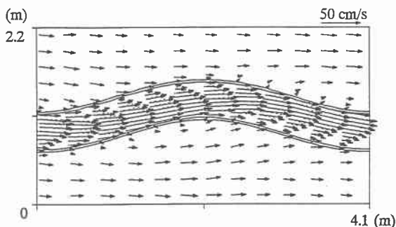
図3 流速ベクトル図（実験） 実線：水面下1cm 破線：水面下6cm
