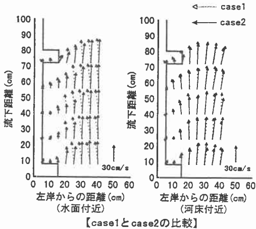
図-4 流速ベクトルの比較(断面 5)
