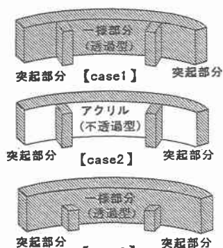
図-1 樹木群水制の構造
