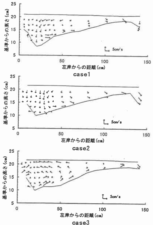
図-5 断面内流速ベクトル(断面 5)
