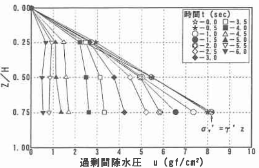
図-2 過剰間隙水圧等時曲線の例
