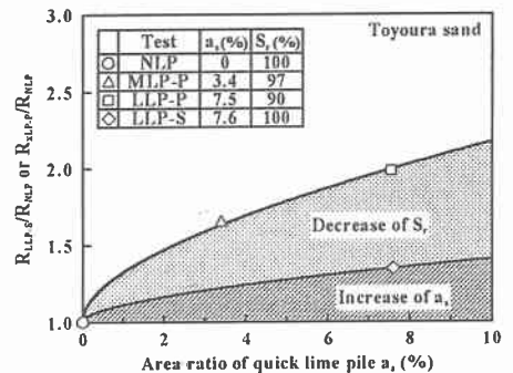
図-5 液状化抵抗比と a_s の関係 (豊浦砂供試体)
