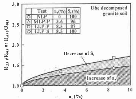
図-6 液状化抵抗比と a_s の関係 (まさ土供試体)
