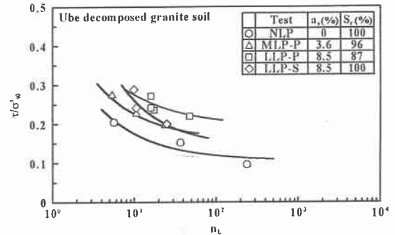
図-4 液状化抵抗曲線 (まさ土供試体)
