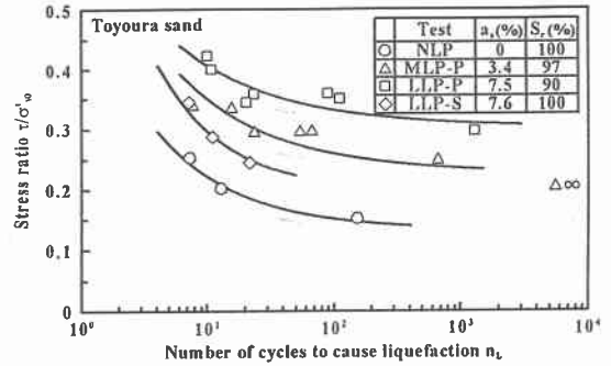
図-3 液状化抵抗曲線 (豊浦砂供試体)
