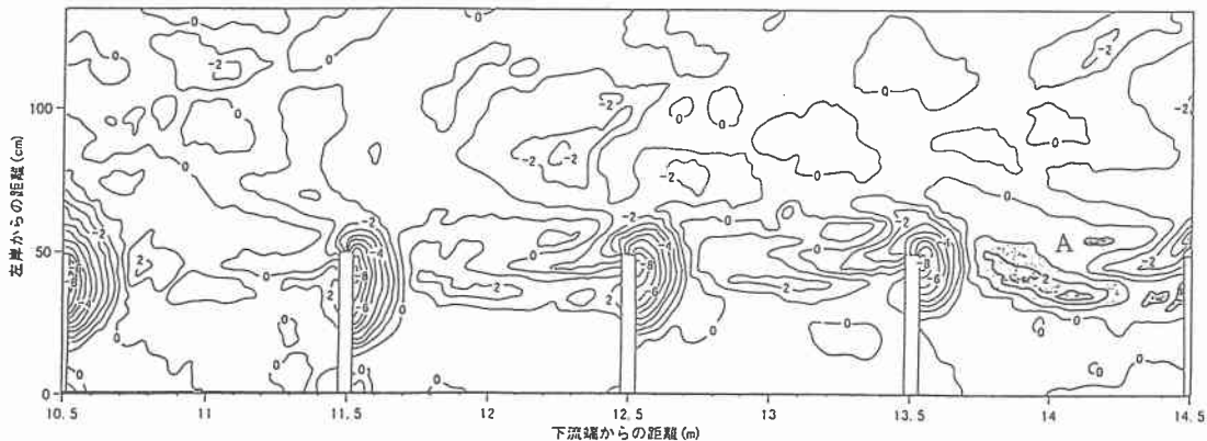
図-1 河床変動コンター（2時間後,実験2）
