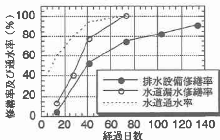
図-3 水道と配水設備の修繕率の変化
