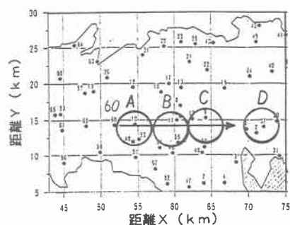
図-4(2) 空間平均を行った範囲
