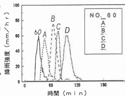
図-4(3) 空間平均した降雨波形の変動
