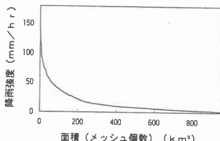
図-3(2) メッシュ毎の降雨強度の大きさ
