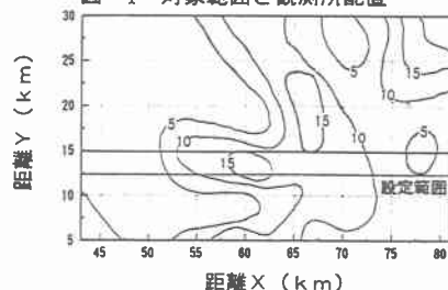
図-2 10分最大雨量コンター図
