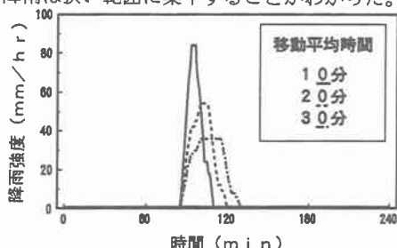
図-3(1) 降雨強度の変動
