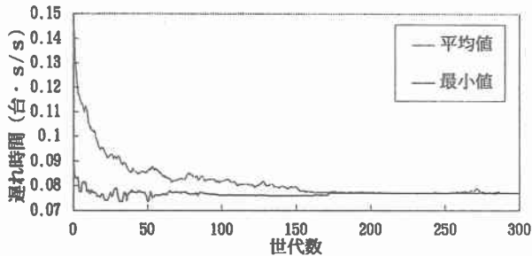
Fig. 2 GAの収束状況
