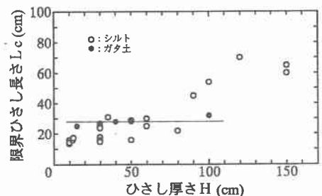
図. 4 ひさし厚さとひさし長さ
