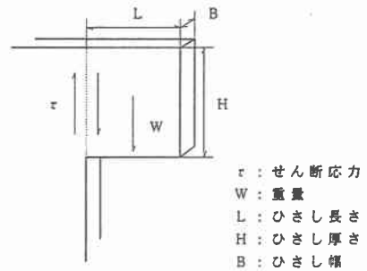
図. 3 ひさし形状
