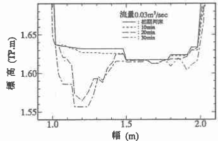
図. 2 横断形状 (中央)
