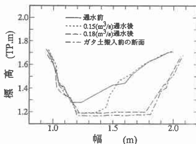
図. 1 横断形状 (下流端)
