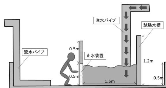
図-2 実験概要（静水時）
