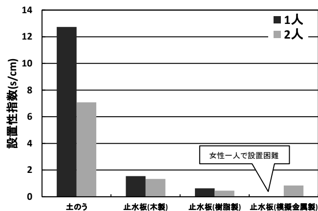
図-1 止水装置設置性指数
