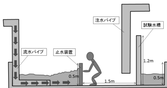
図-4 試験概要（流水時）
