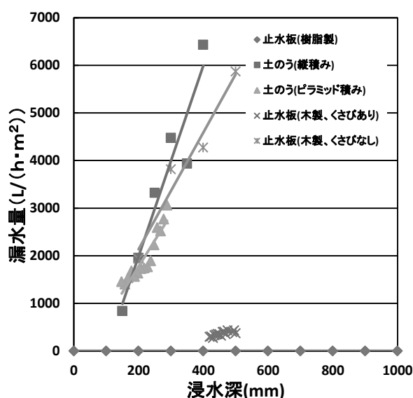
図-3 各止水装置の漏水量（静水時）
