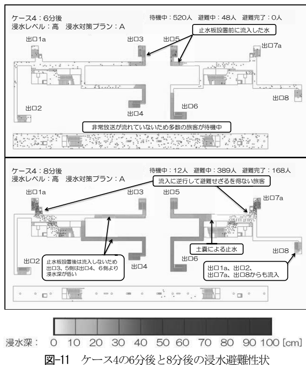
図-11 ケース4の6分後と8分後の浸水避難性状
