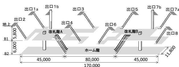
図-7 モデル駅の模式図
