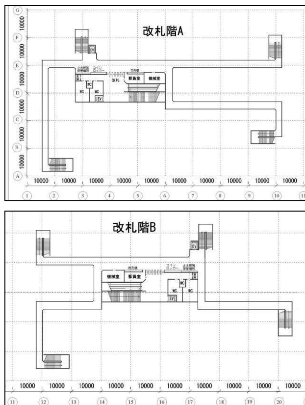
図-8 改札階の平面図
