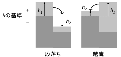
図-4 段差部の水位と適用式
