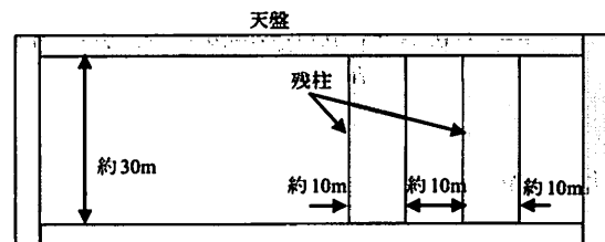
図-3 断面模式図（A-B断面） 4)
