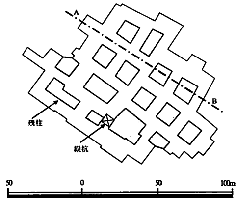
図-2 地下空間形状の一例 4)
