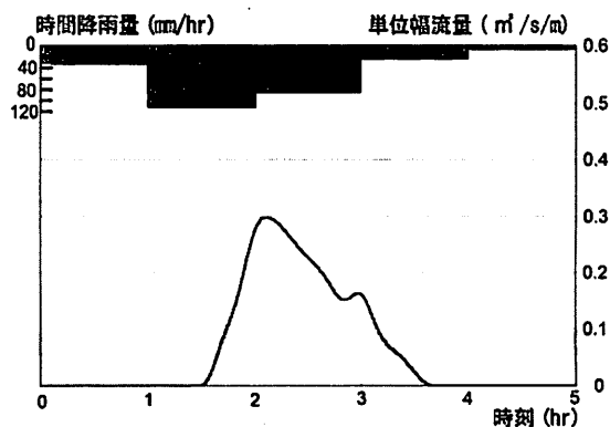
図-10 単位幅流入流量ハイドログラフ
