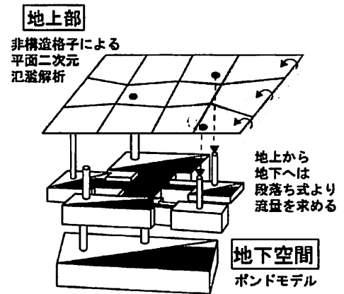
図-1 統合型モデル概念図
