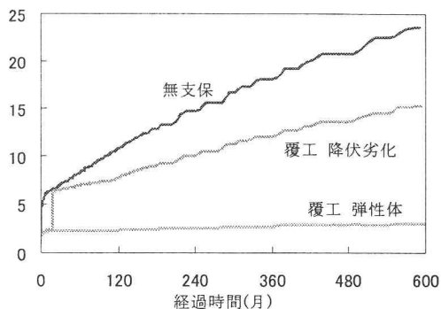
図-12 内空変位の経時変化(覆工状態変化)
