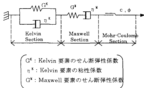
図-9 粘弾塑性モデル
