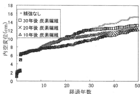
図-14 補修後の内空変位変化(炭素繊維シート工) 表-2 最終変位量と補修コスト
