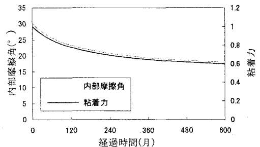
図-11 せん断強度低下の経時変化
