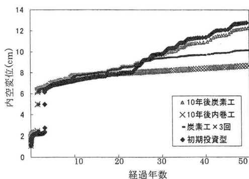
図-15 補修後の内空変位変化(繰り返し補修など)
