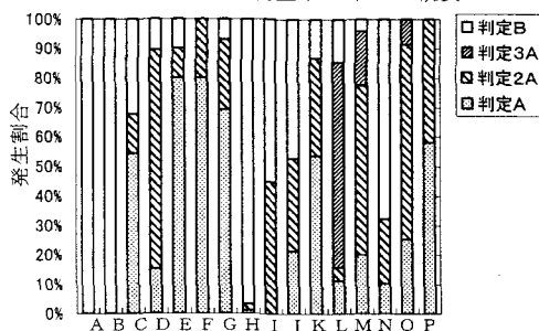
図-6 覆工背面空洞発生割合と経過年数
