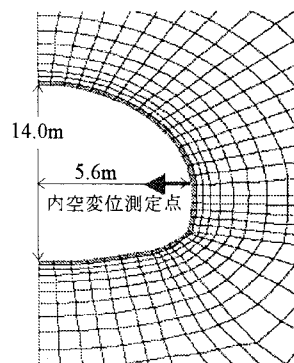
図-10 シミュレーションモデル
