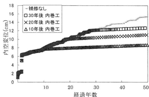
図-13 補修後の内空変位変化(内巻工)
