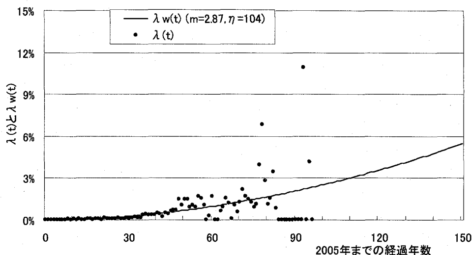
図4 全管種合計の \lambda(t) と \lambda w(t)
