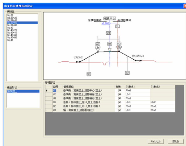
図-18 出来形管理の設定画面
