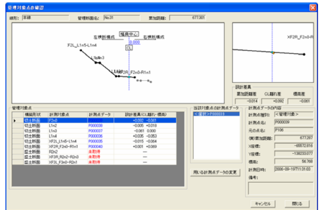
図-21 管理対象点の確認画面
