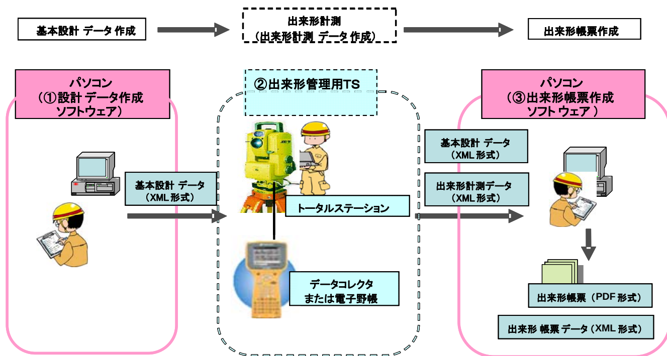
図－１ TS による出来形管理の流れ
