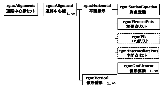
図-5 道路構造物情報(道路中心線セット)
