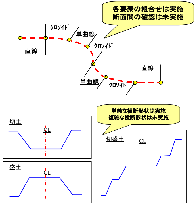
図-13 サンプルデータのチェック内容
