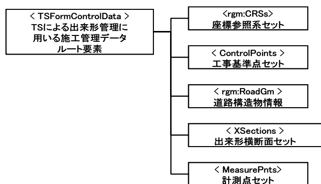
図－２ データ交換標準の全体構成図
