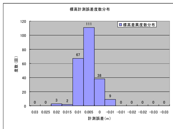
図－10 出来形計測時の標高誤差分布
