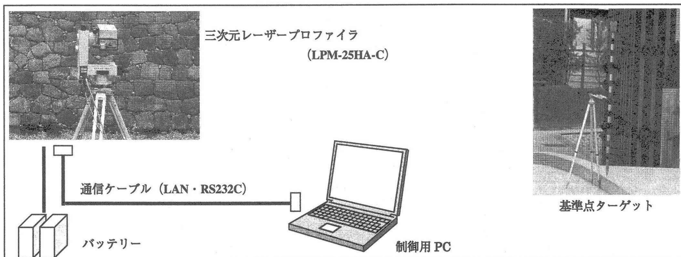
図-1 現地計測機器構成
