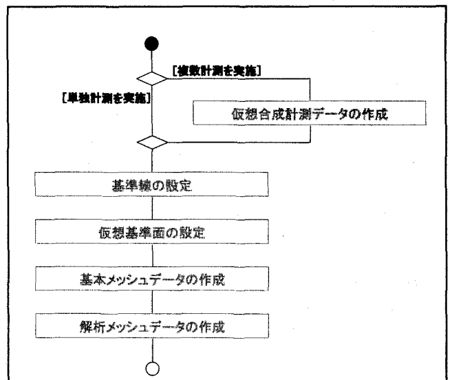
図-8 石垣面の形状解析フロー
