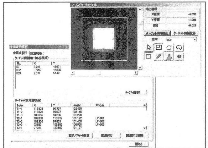
図-5 基準ターゲット座標値の抽出
