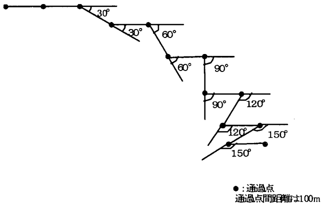
図-2 通過点の設定モデル(1)
