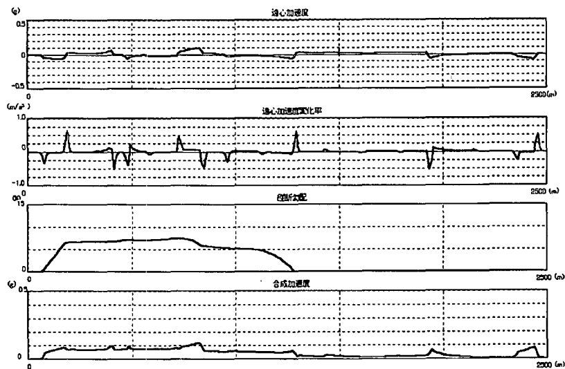
図-8 パラメトリック曲線による3次元道路線形の評価例
