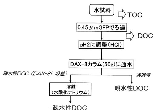
図1. 分画試験操作の概要
