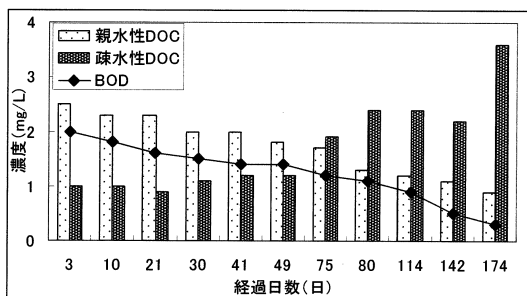
図2. 疎水性及び親水性DOC濃度の経時変化
