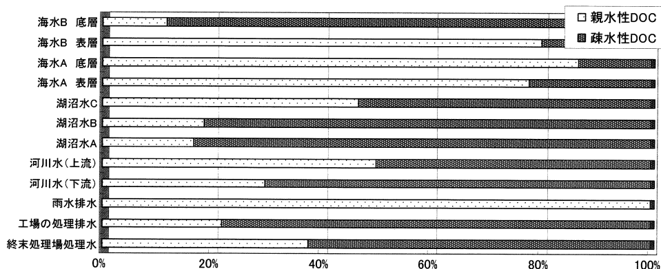
図3. 様々な環境水中の分画試験結果
