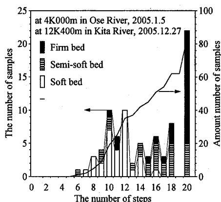
図-2(a) 足踏み回数と河床状態
