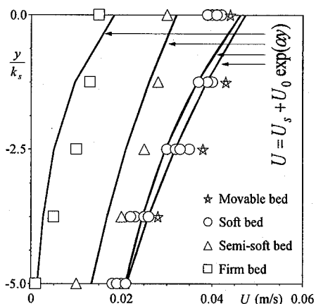
図-8 河床内流速分布
