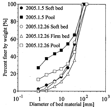
図-3 計測で得られた粒度分布
