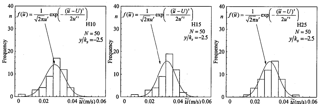
図-7 同一高さにおける異なるケースの \tilde{u} のヒストグラム
