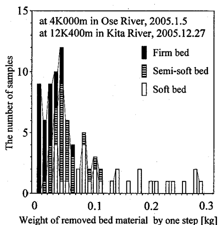
図-2(c) 足踏み1回当たり掃流質量
