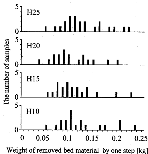
図-5 室内実験における足踏み1回当たりの掃流砂質量
