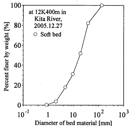
図-4 足踏みによって流出した河床材料の粒度分布
