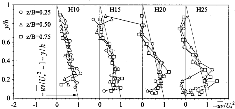
図-9 レイノルズ応力分布
