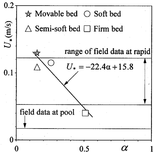
図-10 係数 \alpha と摩擦速度 U_* の関係
