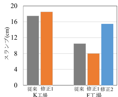
図-6 スランプ試験結果
