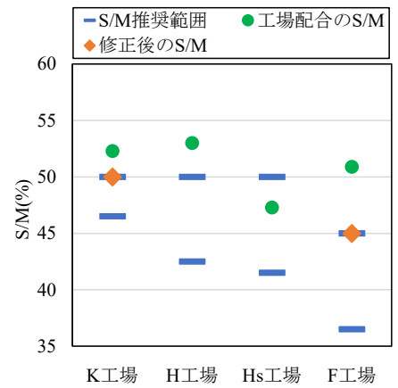
図-4 各工場のS/MとS/M推奨範囲
