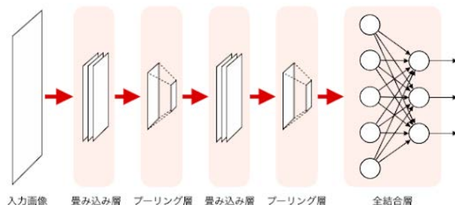
図 1 CNN 概要
