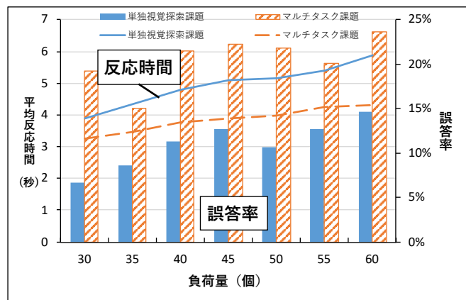
図 2 視覚探索の平均反応時間と誤答率
