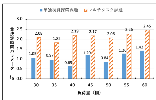
図 5 視覚探索の非決定時間パラメータ t_0 比較
