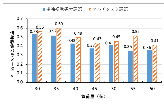
図 4 視覚探索の情報収集パラメータ v 比較
