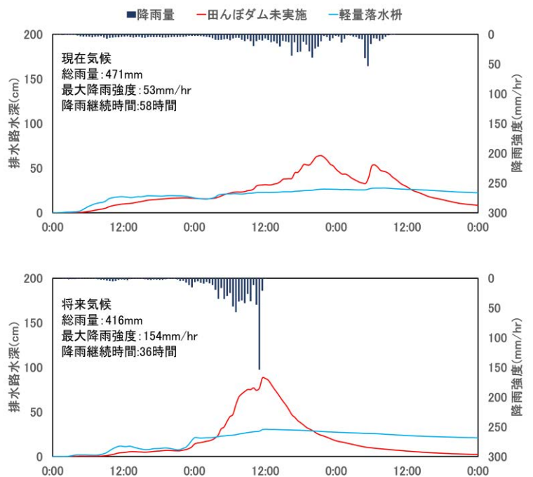
図-2 排水路水深の時間変化
