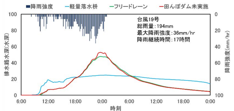
図-1 台風 19 号を対象とした排水路水深の時間変化
